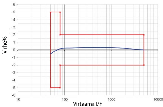
Tyypillinen virhekkäyrä Q3 4 R80H
