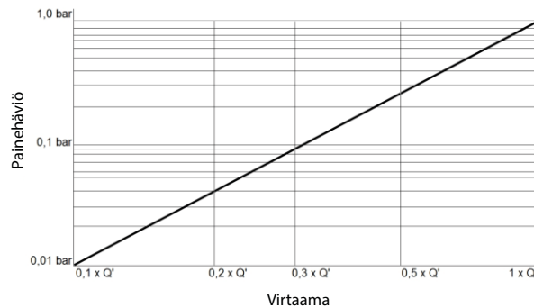
Typillinen painehäviökäyrä
